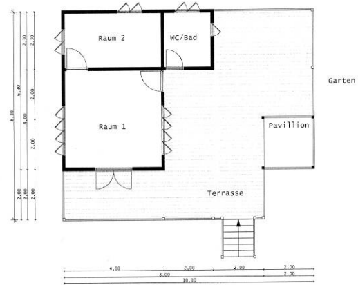
Thai House Grundriss EG
